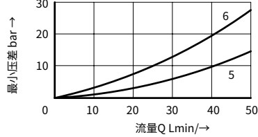
\Delta p_{min} - q_v 特性曲线
