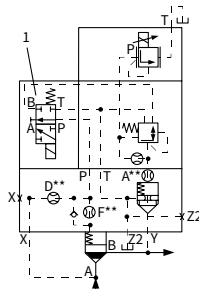
LFA..DREWW-7X/006 NG 63
