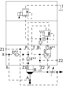
LFA..DREZ-7X/014 NG 63
