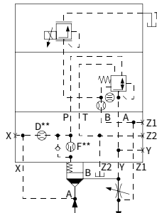
LFA..DREZ-7X/014 NG 40, 50
