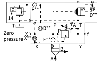
LFA..DBEM-6X/... NG 80, 100
