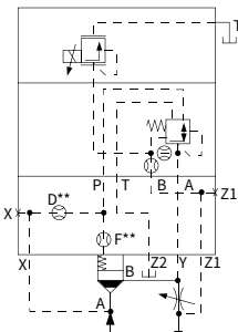
LFA..DREZ-7X/014 NG 25, 32
